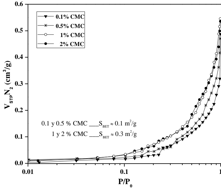
Figura 5. Isotermas de adsorción de N_2 a 77K de las esponjas cerámicas
